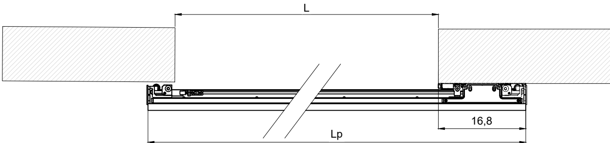
TLOCRT
