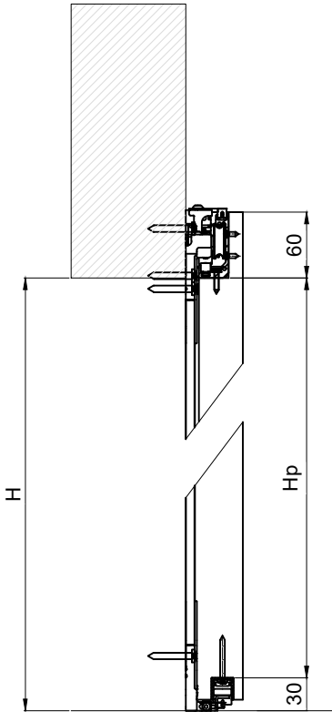
PRESJEK
